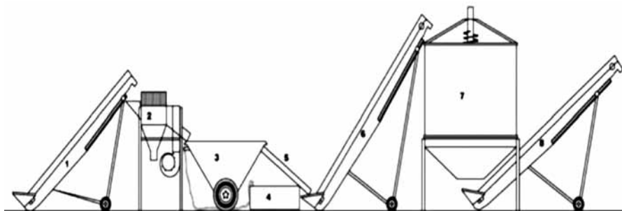
1-5-6-8 კონვეიერი, 2-სეპარატორი, 7 — საშრობი, 3-4 შემკრები ბუნკერი
